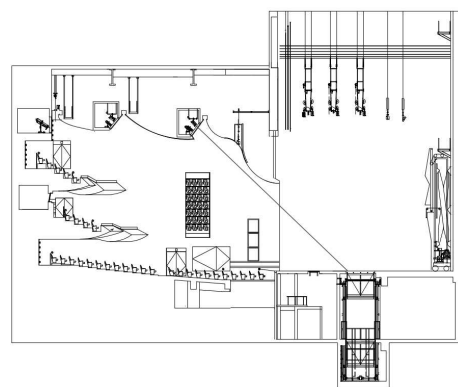
舞台断面図
