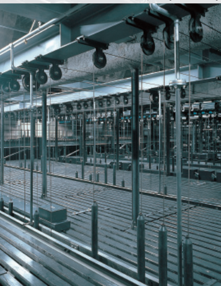
▼作業性を重視した舞台上部スノコ spacious gridiron above stage
